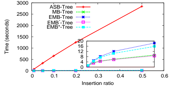
(d) Total update time.
